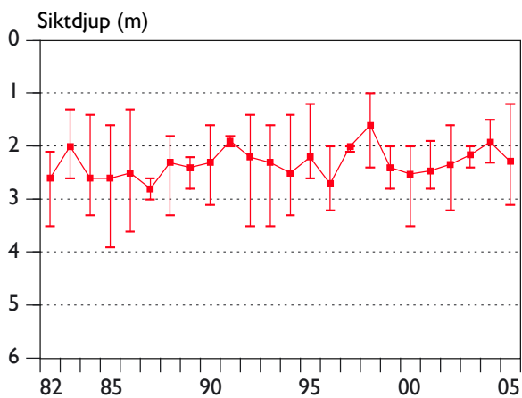
Figur 6. Siktdjupet i Mariestadsfjärden vid station M2 1982-2005. Medel-, min- och max-värden anges för resp. provtagningssäsong.
