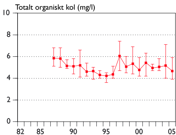
Figur 10. Mängden organiskt material (uttryckt som TOC) i Mariestadsfjärdens ytvatten (0,5 m) vid station M2 1986-2005. Medel-, min- och max-värden anges för respektive säsong.
