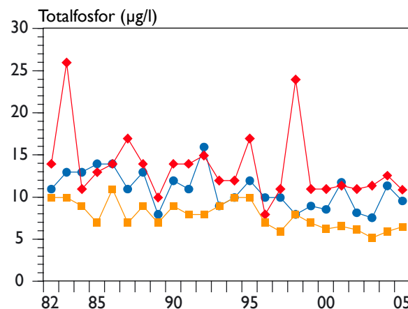
Figur 5. Totalfosforhalt i ytvatten (0,5 m) vid M1 och M2 i Mariestadsfjärden, samt vid Dagskärsgrund i Storsjön. Samtliga data är medelvärden för resp. provtagningssäsong 1982-2005. Symboler enligt figur 3.
