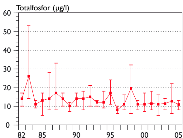
Figur 4. Totalfosforhalt i Mariestadsfjärdens ytvatten (0,5 m) vid station M2 1982-2005. Medel-, min- och maxvärden anges för resp. provtagningssäsong.
