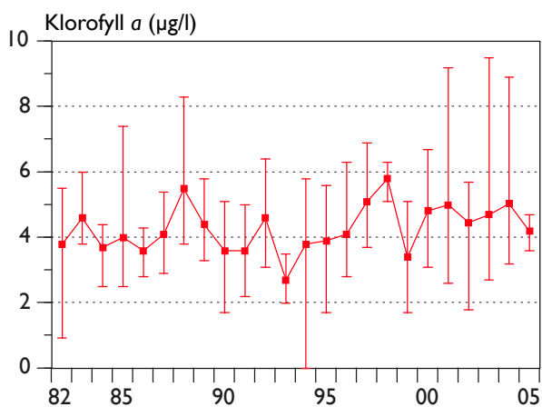
Figur 8. Klorofyllhalt i Mariestadsfjärdens ytvatten (0,5 m) vid station M2 1982-2005. Medel-, min- och max-värden anges för resp. provtagningssäsong.
