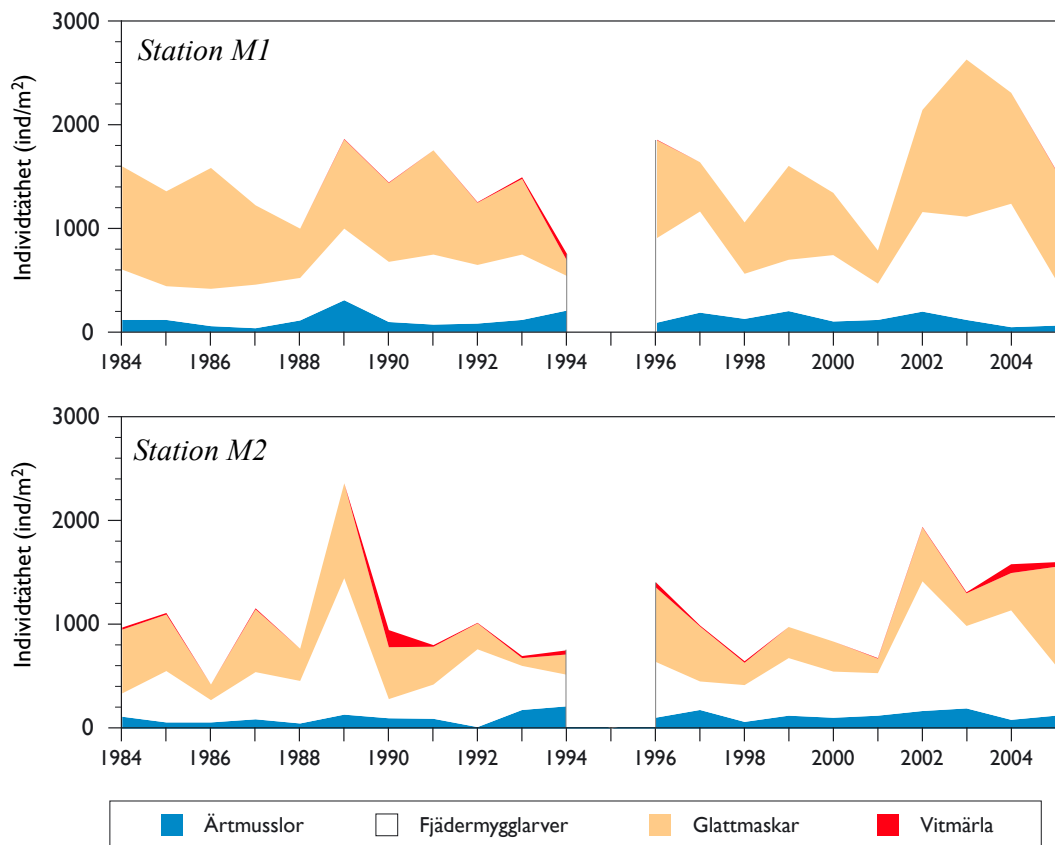
Figur 12. Individtätheter (individer/m 2 ) för de fyra vanligaste djupbottentaxa vid M1 och M2 i Mariestadsfjärden 1984 – 2005. Data från maj 1984 – 1994, samt oktober 1996 – 2005.
