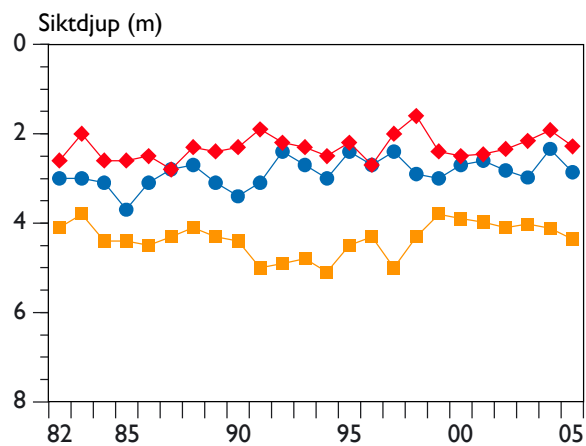
Figur 7. Siktdjupet vid M1 och M2 i Mariestadsfjärden, samt Dagskärsgrund i Storvänern. Samtliga data är medelvärden för resp. provtagningssäsong 1982-2005. Symboler enligt figur 3.
