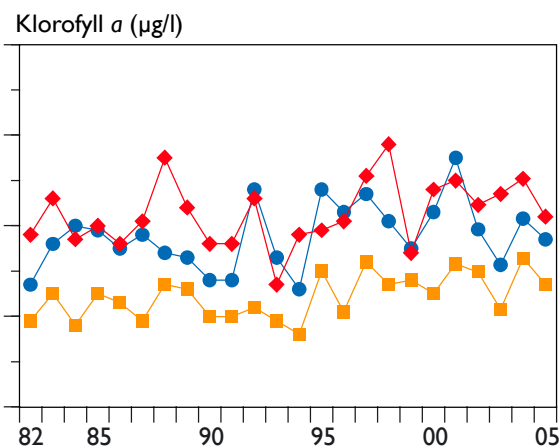
Figur 9. Klorofyllhalt i ytvatten (0,5 m) vid M1 och M2 i Mariestadsfjärden, samt vid Dagskärsgrund i Storvänern. Samtliga data är medelvärden för resp. provtagningssäsong 1982-2005. Symboler enligt figur 3.
