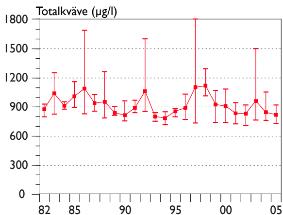
Figur 2. Totalkvävehalt i Mariestadsfjärdens ytvatten (0,5 m) vid station M2 1982-2005. Medel-, min- och maxvärden anges för resp. provtagningssäsong.
