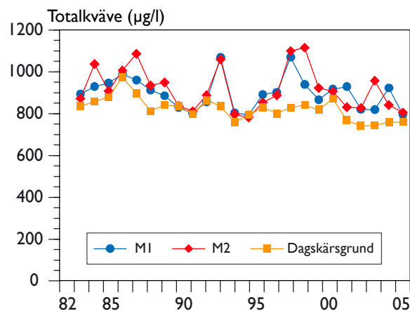
Figur 3. Totalkvävehalt i ytvatten (0,5 m) vid M1 och M2 i Mariestadsfjärden, samt vid Dagskärsgrund i Storsjön. Samtliga data är medelvärden för resp. provtagningssäsong 1982-2005.
